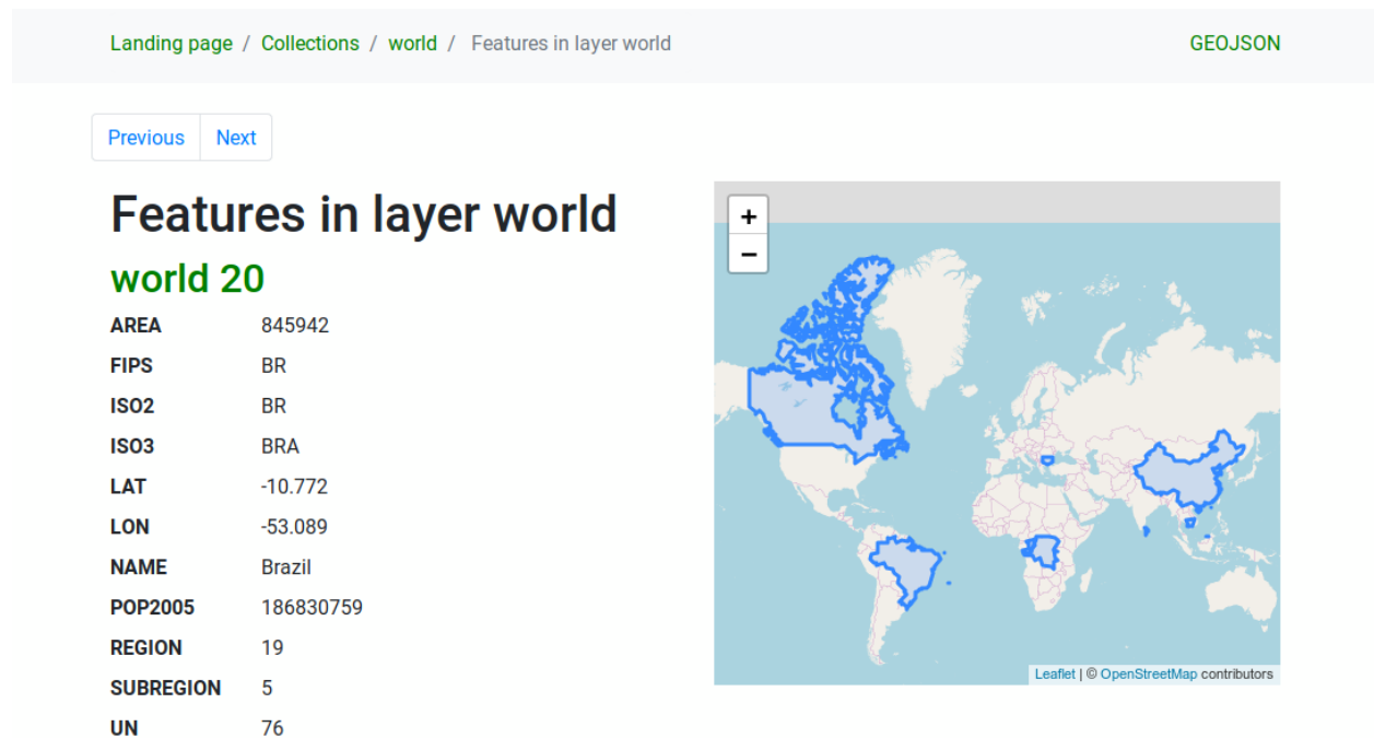
그림 3.27: 서버 OAPIF 피처 목록 페이지
