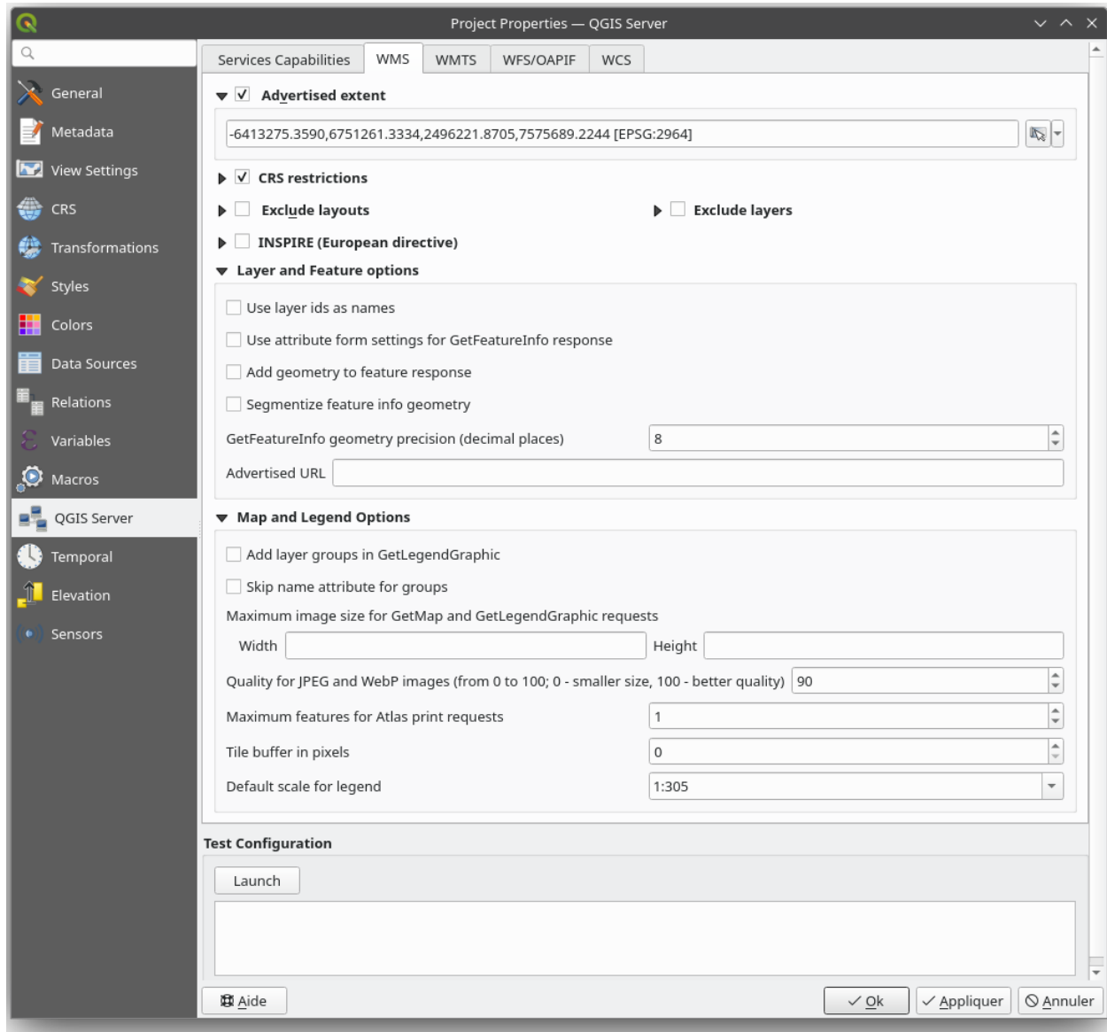
그림 2.3: WMS 탭에서 정의할 수 있는 항목들
