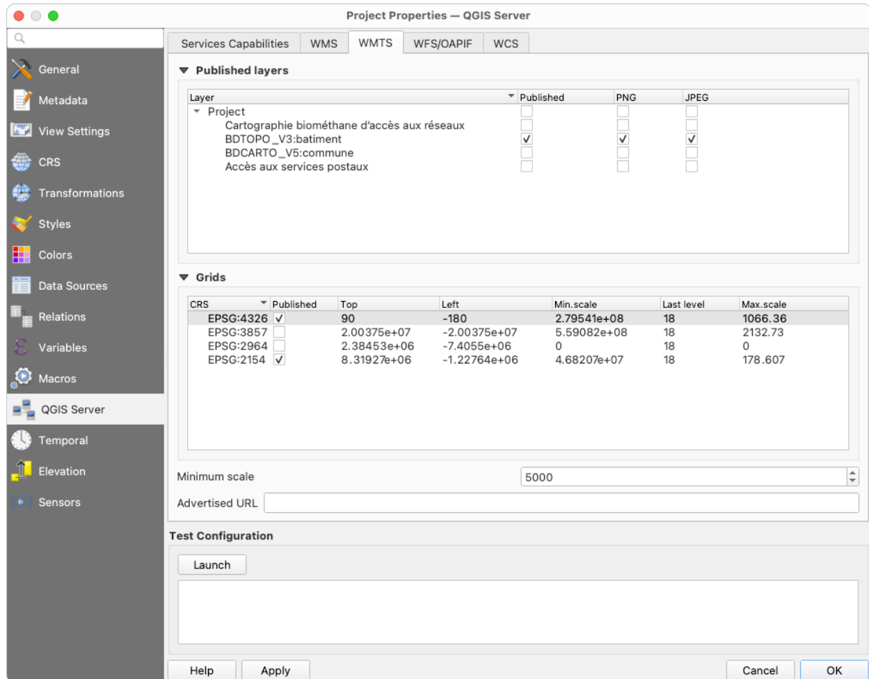
그림 2.4: WMTS 탭에서 정의할 수 있는 항목들
