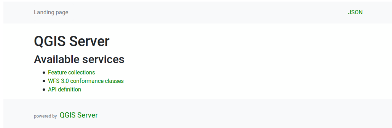
그림 3.24: 서버 OAPIF 랜딩 페이지
