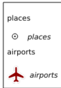
図 3.19: ITEMFONTITALIC=TRUE の凡例
