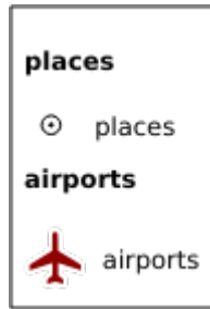
図 3.13: LAYERFONTBOLD=TRUE の凡例
