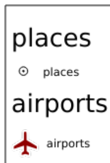
図 3.14: LAYERFONTSIZE=20 の凡例
