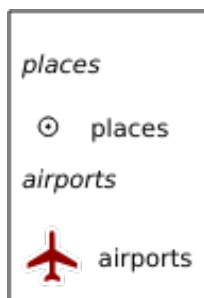
図 3.15: LAYERFONTITALIC=TRUE の凡例
