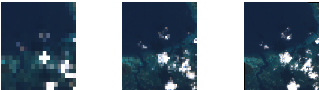
図 3.23: 左から、WIDTH=20&HEIGHT=20、WIDTH=50&HEIGHT=50、WIDTH=100&HEIGHT=100
