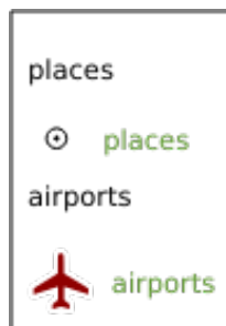
図 3.20: ITEMFONTCOLOR=0x5f9930 の凡例
