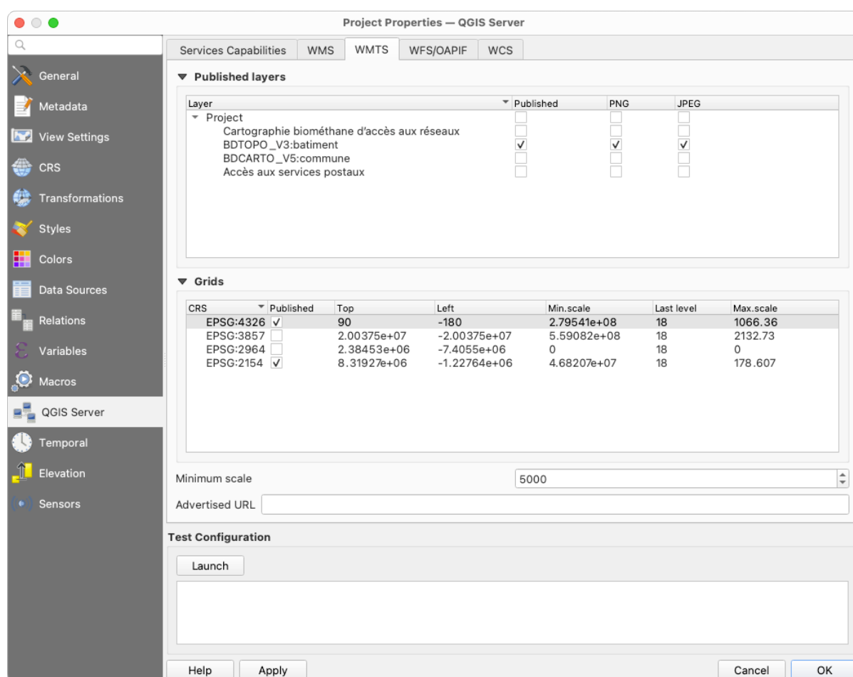
Fig. 2.4: Definizioni nella scheda WMTS
