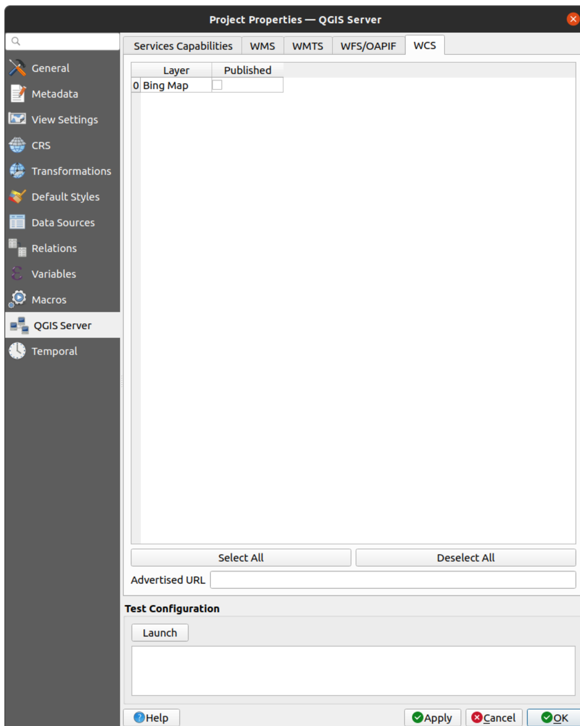
2.6. ábra: Definitions in the WCS tab
