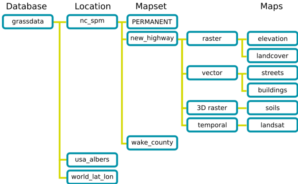
Abb. 12.2: Die GRASS Datenbankstruktur (aus der GRASS Hilfe)
