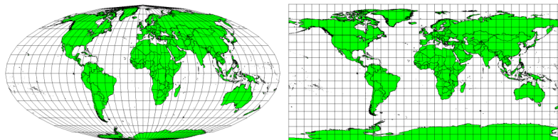
Abb. 9.6: Die Welt in verschiedenen Projektionen. Links eine flächentreue Projektion nach Mollweide, auf der rechten Seite eine Platkarte oder Rektangularprojektion als abstandstreue Zylinderprojektion.
