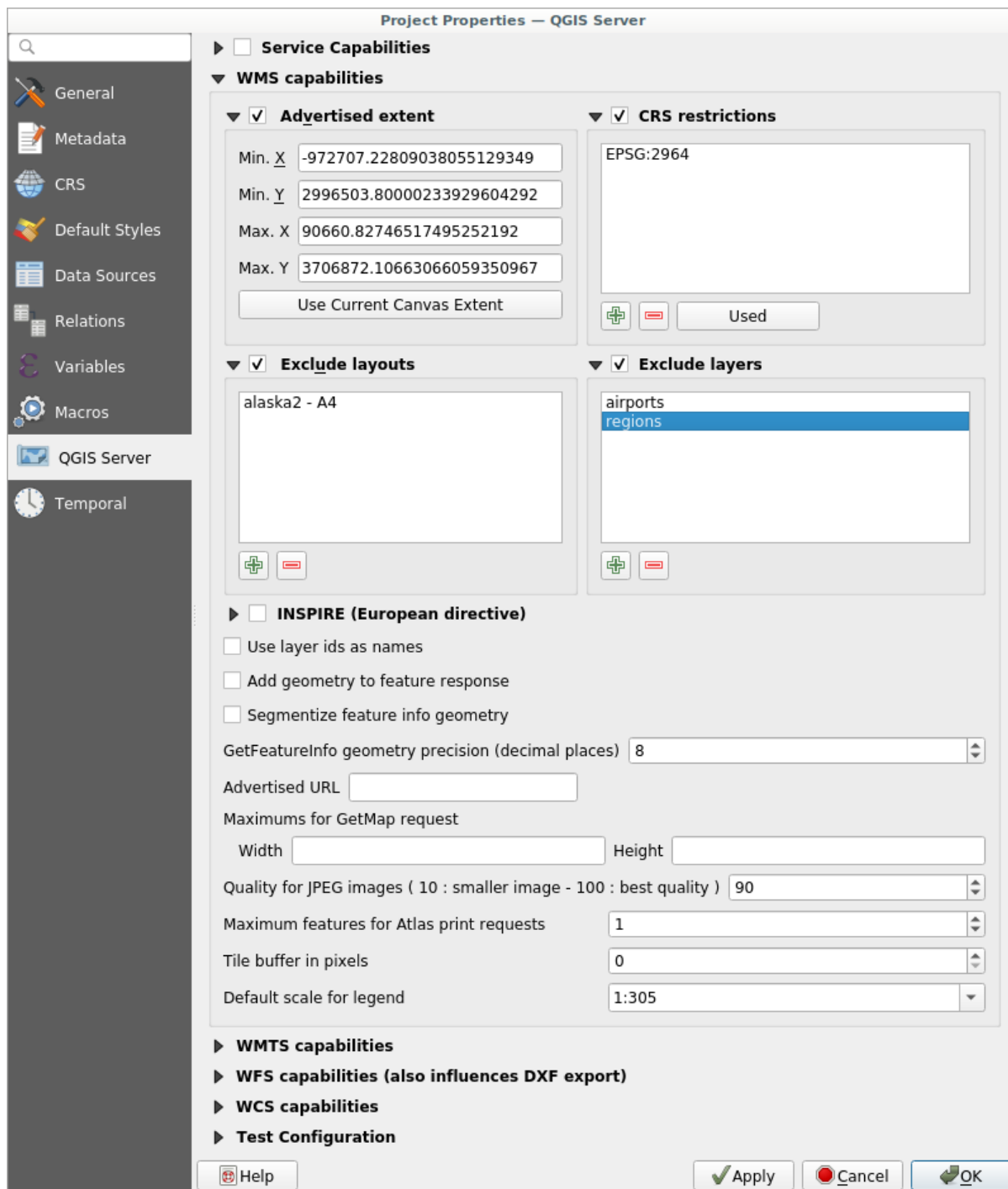
図 2.2: QGIS サーバーの WMS / WFS / WCS プロジェクトの定義
